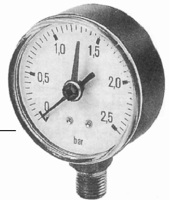
-Figura 1: Manometro 0-2,5 Bar attacco radiale con lancetta rossa.
