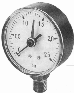
-Figura 1: Manometro 0-2,5 Bar attacco radiale con lancetta rossa.
