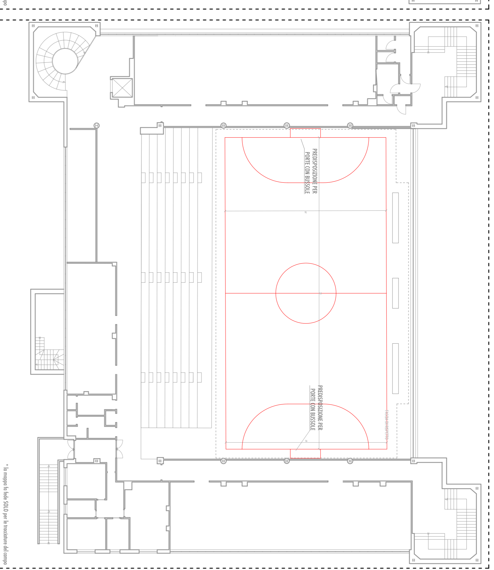
SCHEMA TRACCIATURE CAMPO GALETTO
