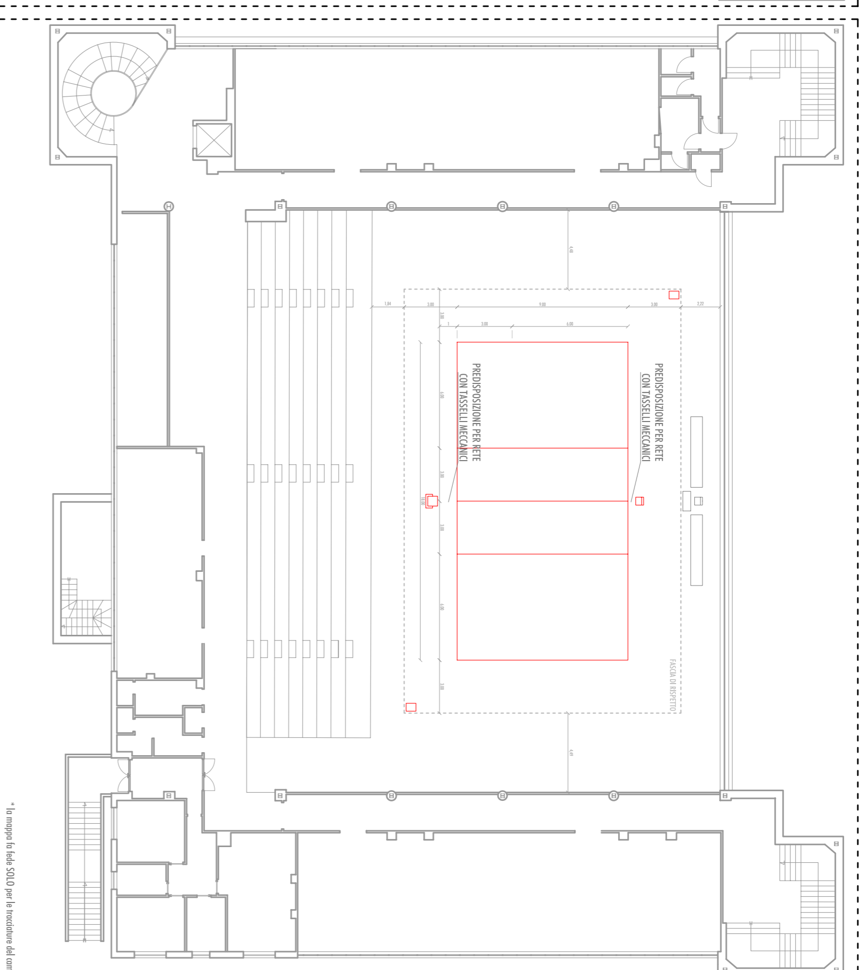
SCHEMA TRACCIATURE CAMPO PALLAVOLO
