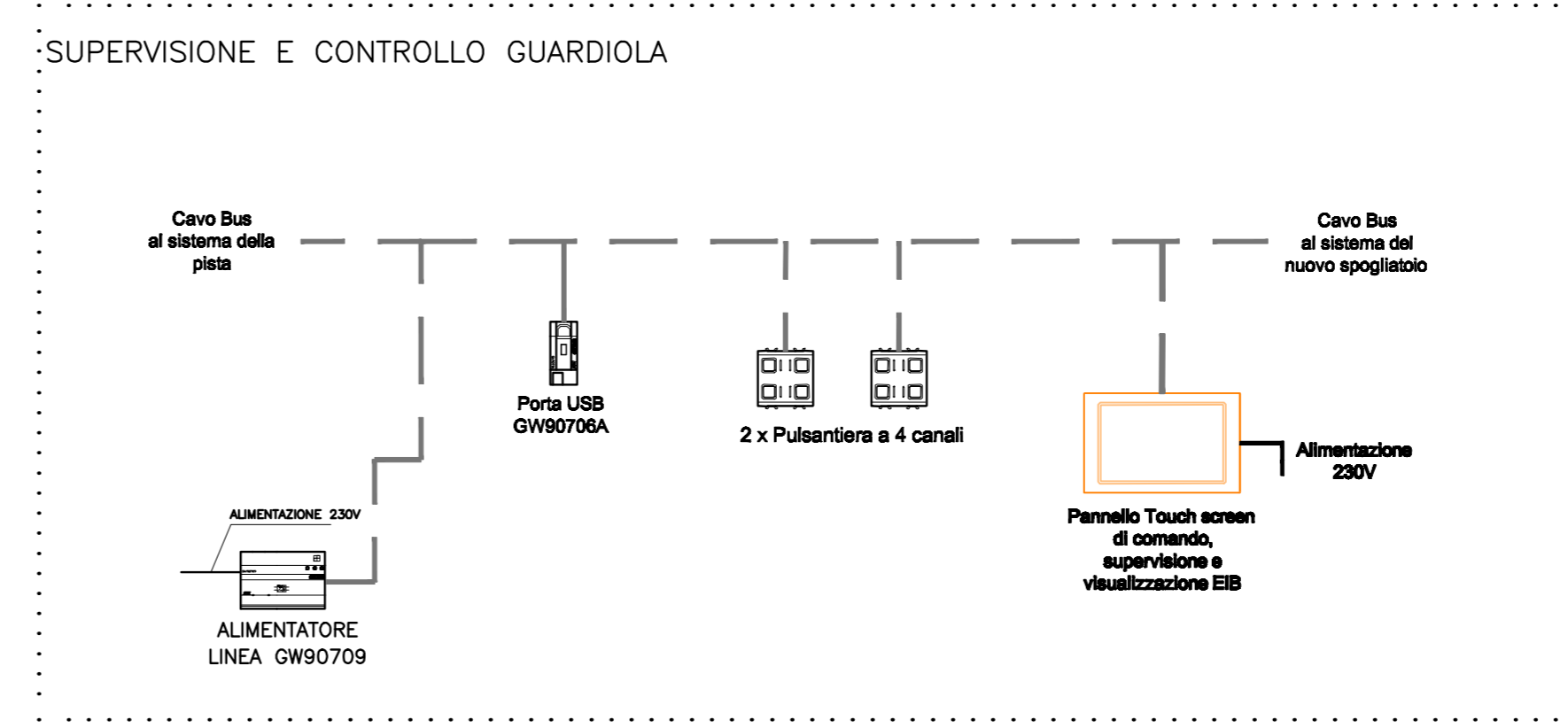
SCHEMA FUNZIONALE
