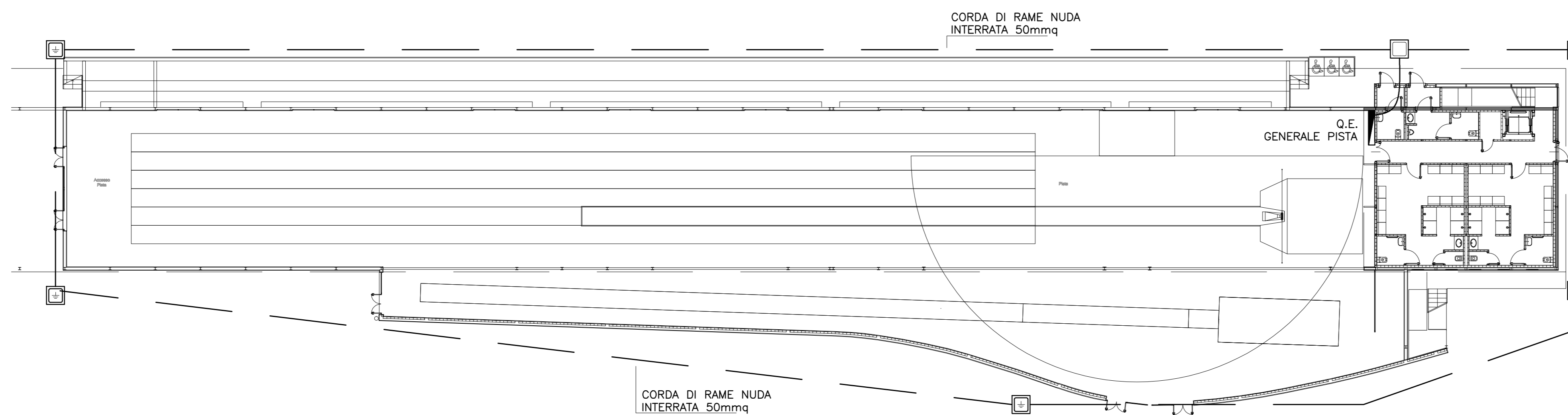
PIANTA PIANO TERRA scala 1:200
