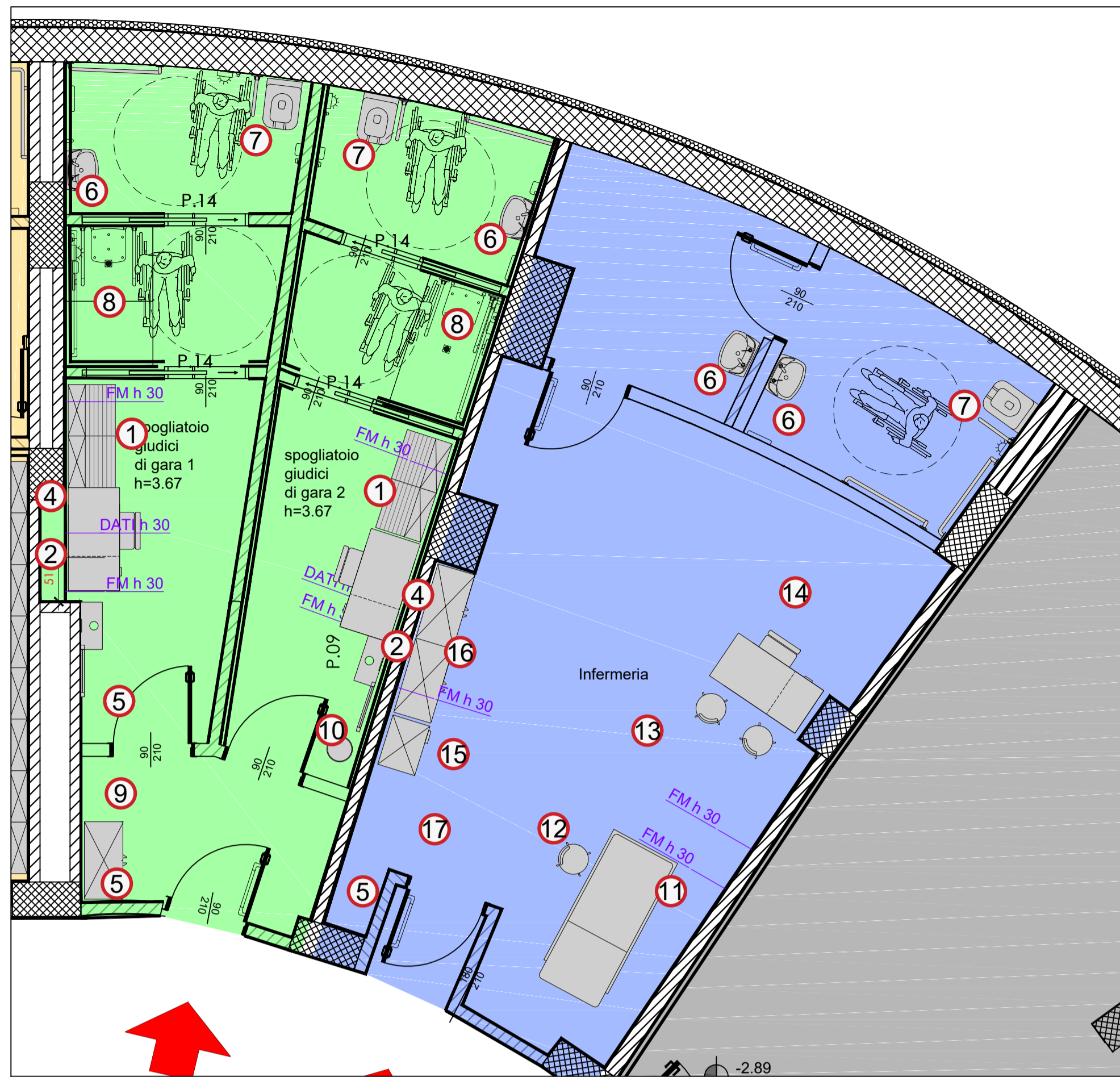
Pianta - scala 1:50
