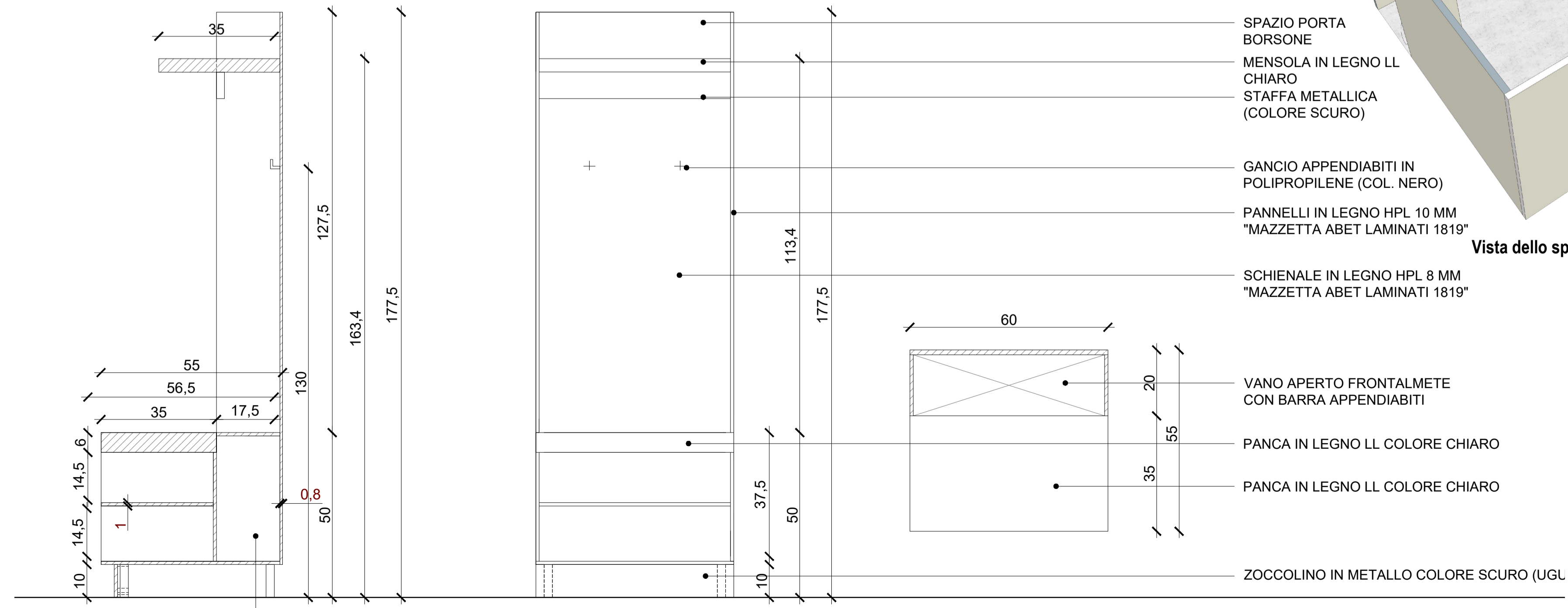
Armadietto spogliatoi - Scala 1:10
