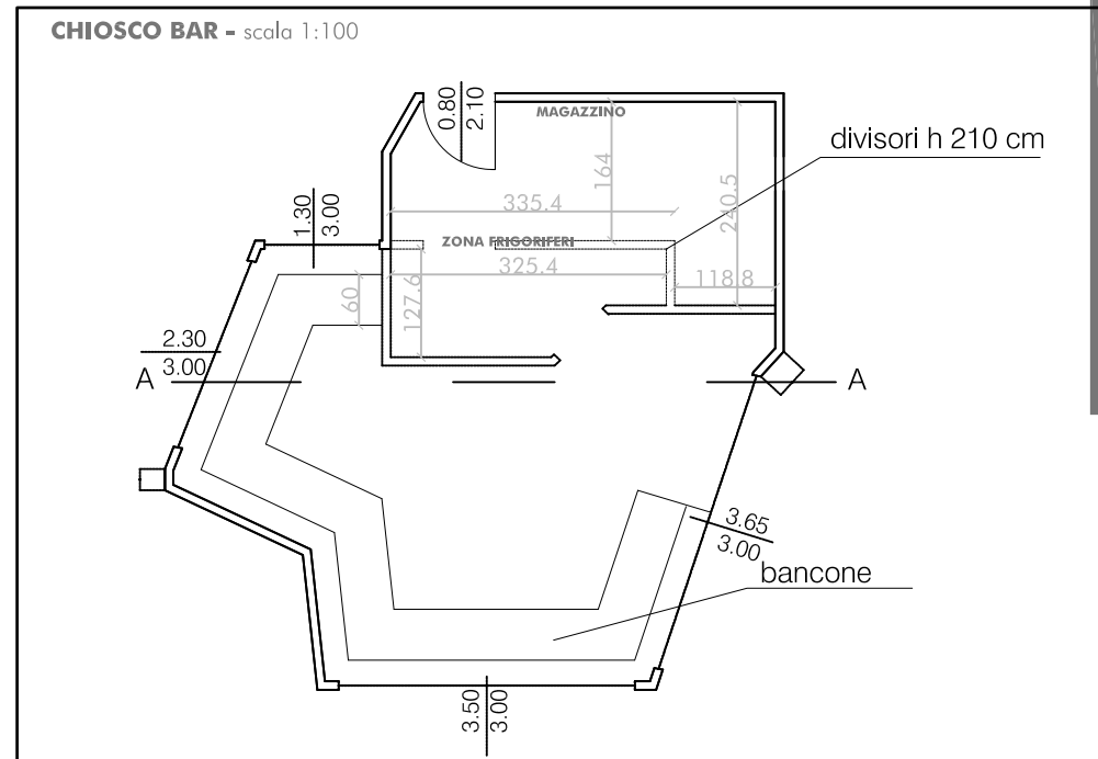
CHIOSCO BAR _ RAPPORTI AERO ILLUMINANTI RISPETTATI _ struttura completamente apribile
