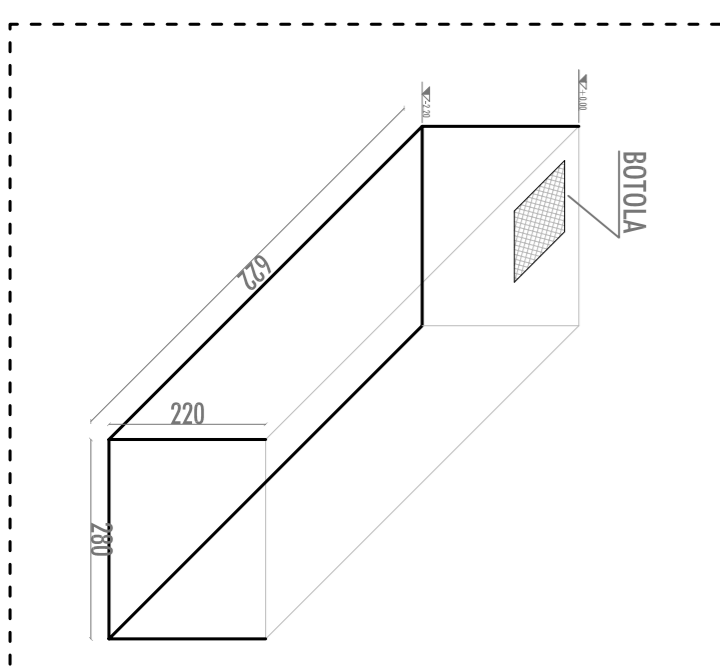
STATO DI FATTO - SCHEMA VASCA DI COMPENSO
